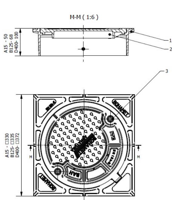
Rys 2. Właz L315 A15/B125/D400.
