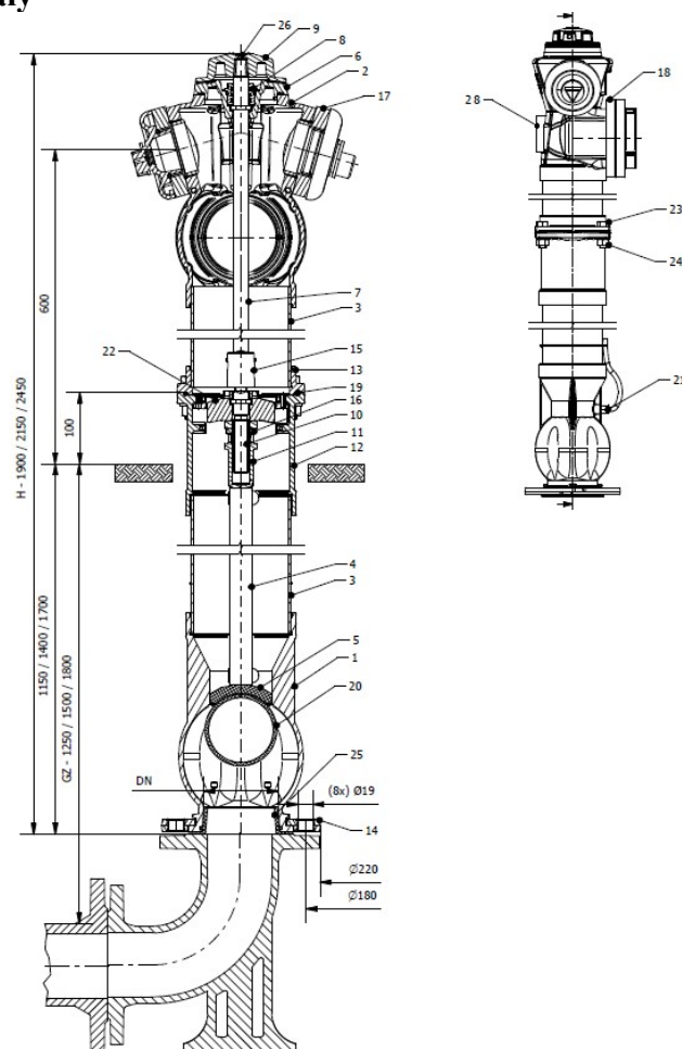
Hydrant HN3-L-PW DN100 z podwójnym zabezpieczeniem kulowym
