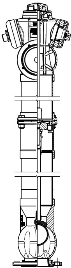
Hydrant zamknięty
